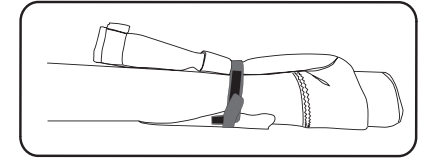
図11: セイルを巻いた後、パッドを折り曲げ、タックベルトでセイルとパッドを一緒に巻き、ベルクロで留める。
