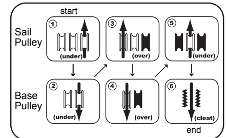
図13: Chinookタイプのエクステンションのブーリーへのラインの通し手順
