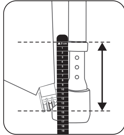
図8: タックベルトのメジャーを使用し、マストのボトムからダウンホールブーリー中央ボトムまでの長さを図ります。
